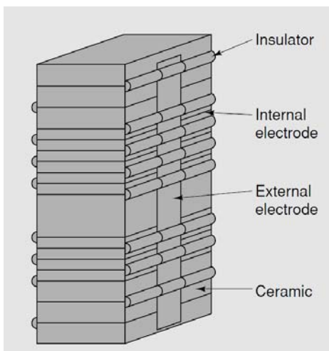
그림 2 적층형 압전 액추에이터의 구조 [17] Fig. 2 Structure of Piezoelectric Stack Actuator [17]
