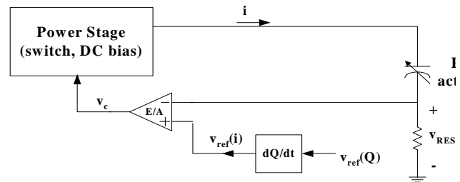
b) 전하량 기준치를 미분한 차지제어 방식 b) The charge control method using differentiation of the charge reference
