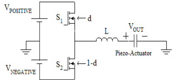
그림 1 마이크로 변위제어 시스템 내의 압전 액추에이터 구동을 위한 클래스 D급 스위칭 증폭기
