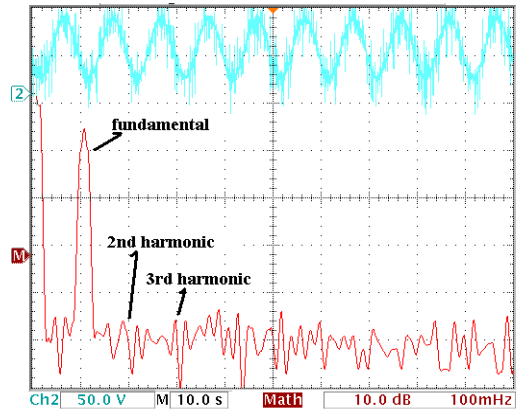
a) 압전 전압의 시간 및 주파수 영역의 파형 a) Piezo-voltage swing and the FFT waveforms
