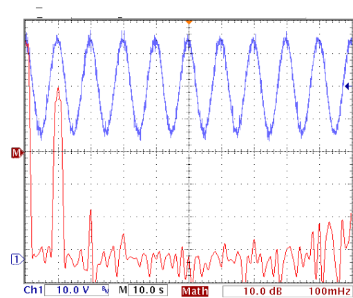
b) 변위 (21-38um) 및 푸리에 변환 파형 b) Displacement (21-38um) and the FFT waveforms
